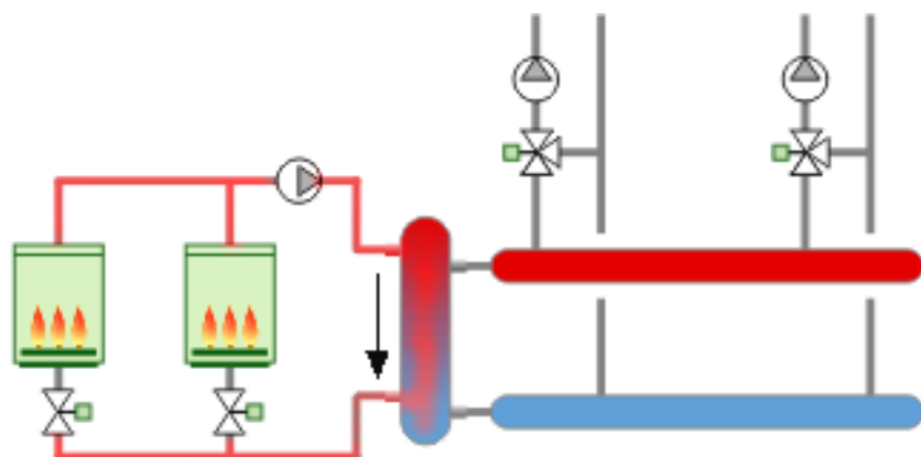
Schéma défavorable à la condensation
